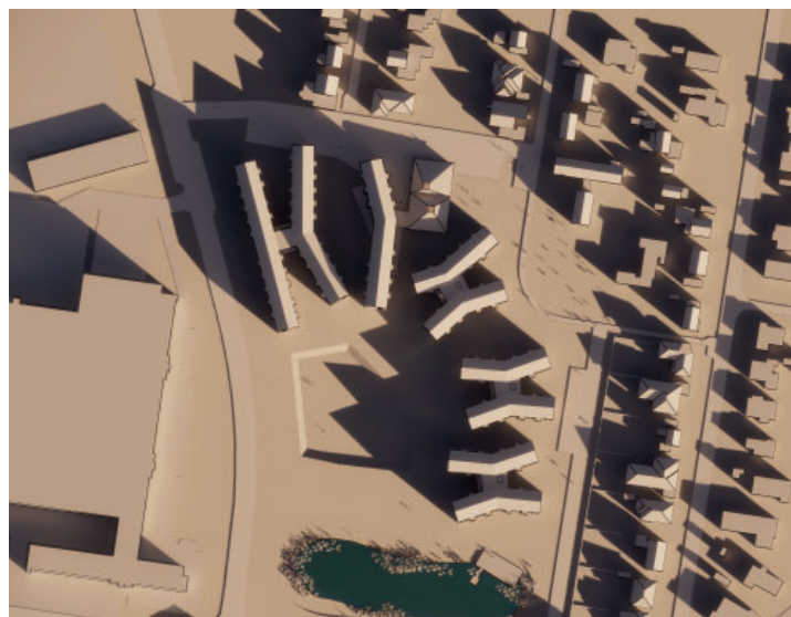
21. december kl. 08:00
