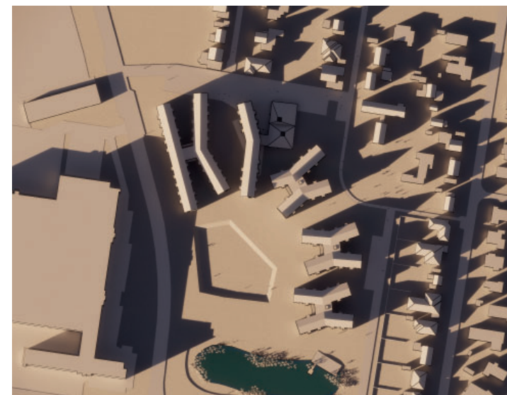
21. december kl. 16:20
